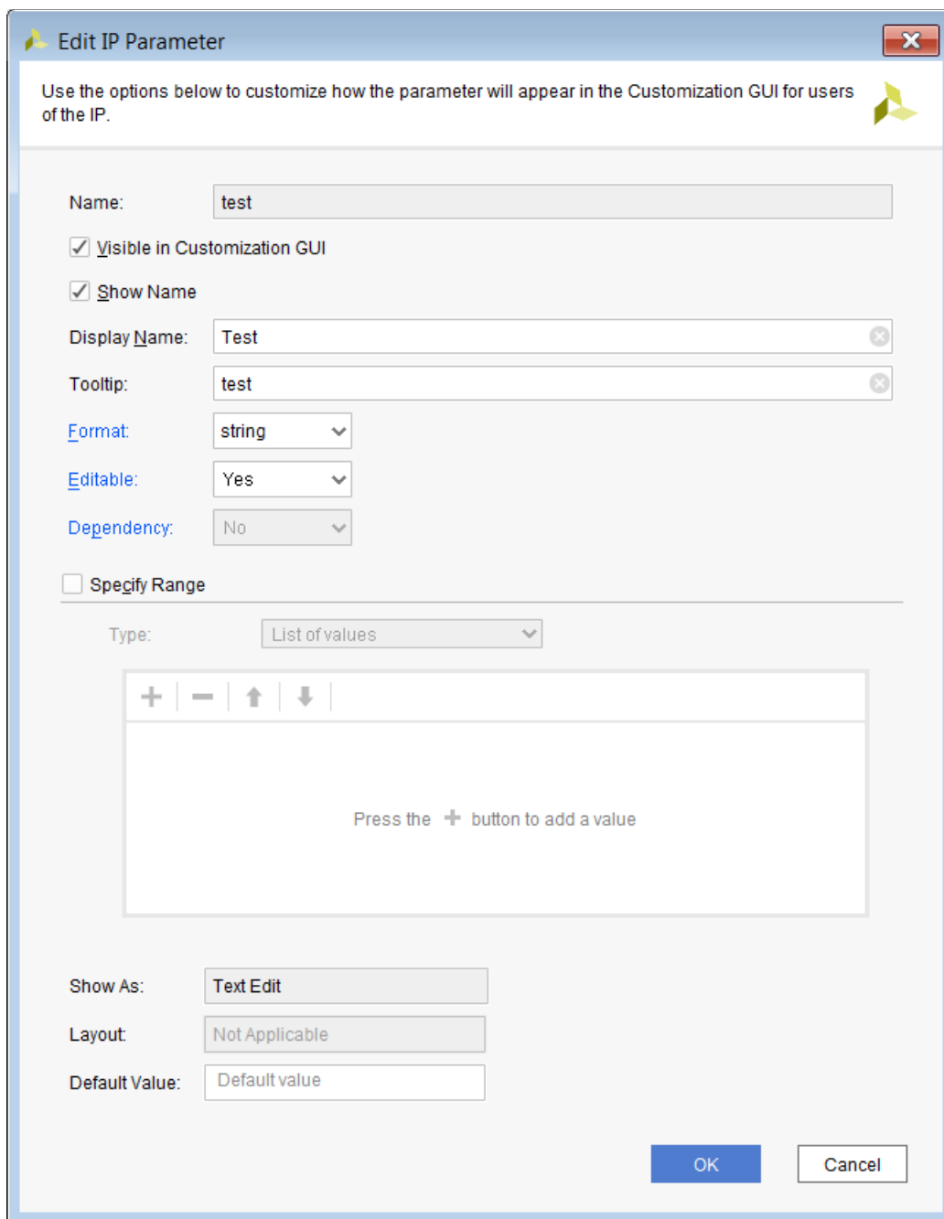
Figure 4-10: Edit IP Parameter
