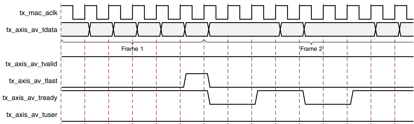
Figure 3-41: TX AV Traffic Timing
