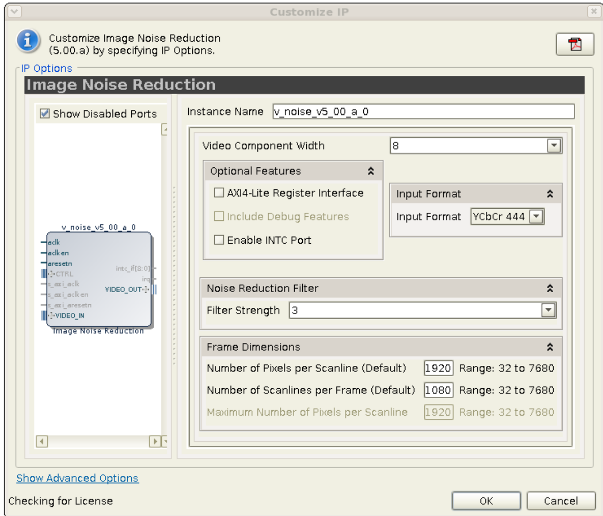
Figure 5-1: Vivado IP Catalog GUI
